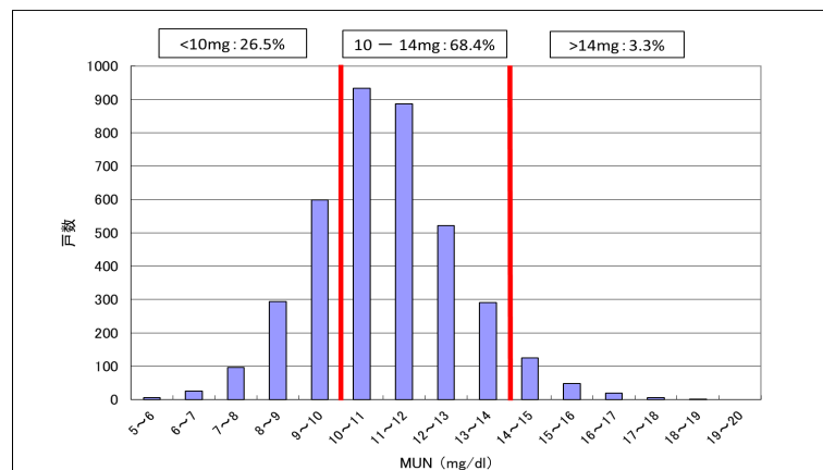
図2 2019年度 個乳年間平均MUNの分布
